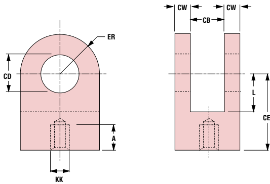
Plain Rod Clevis
